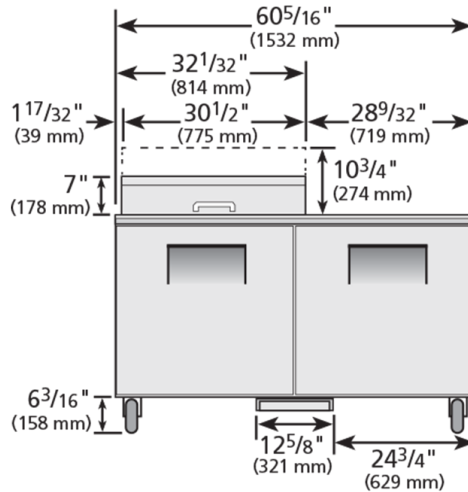
ELEVATION
